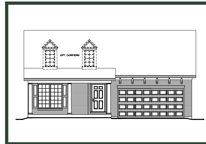
Elevation A
